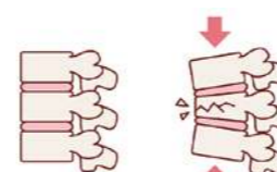
図3 椎体
