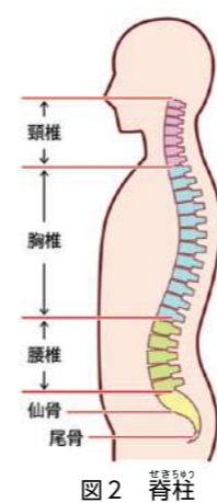
図2 脊柱
